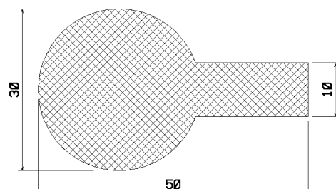
25793 NBR/hg/ 8069
